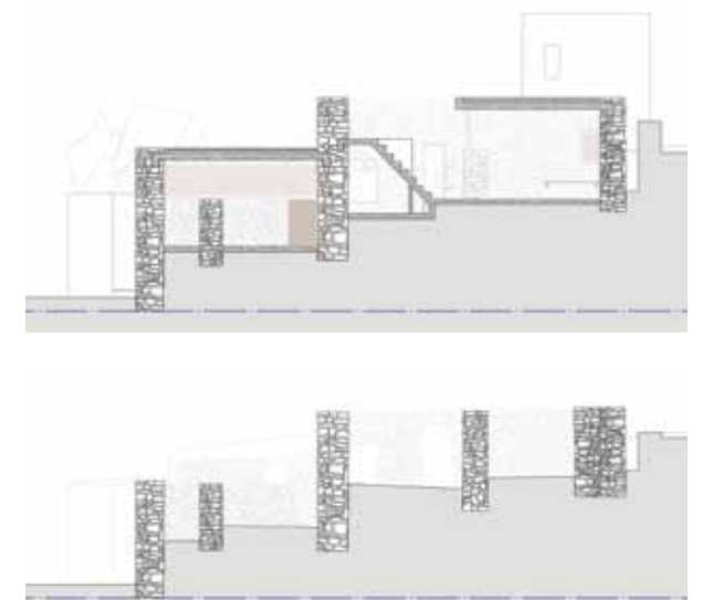
Τομές
